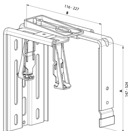
KBT4/1 (B=116-169; A=147-524) KBT4/2 (B=170-227; A=147-524) (pour boîtier 56x58)
