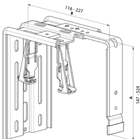
KBT3/1 (B=116-169; A=147-524) KBT3/2 (B=170-227; A=147-524) (pour boîtier 56x58)
