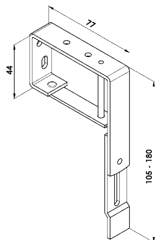
KBT1 (pour boîtier 40x40)
