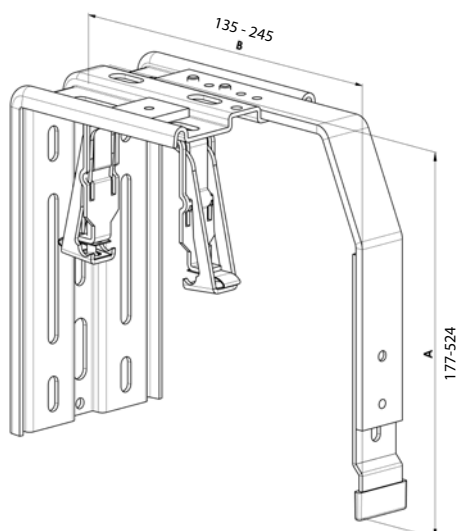
KBT5/1 (B=135-190; A=177-524) KBT5/2 (B=191-245; A=177-524) (pour boîtier 56x58)
