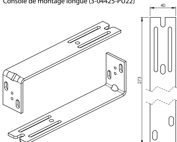
Console de montage longue (3-04425-PU22)
