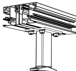
Placement de console élevée au milieu
