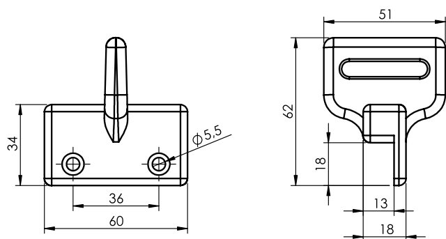
Équerre supérieure SB – Alu
