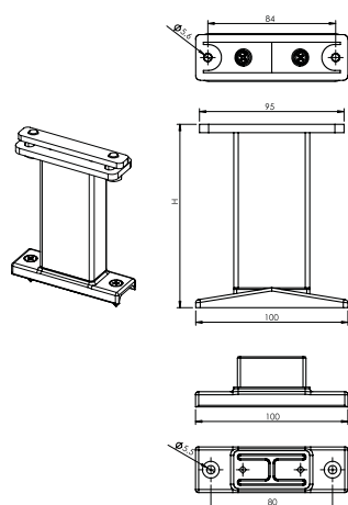
Équerre de coulisse VL Av (2-01410-PU11X)
