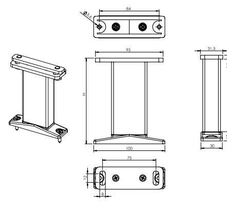
Équerre de coulisse VL Cv (2-01412-PU11X)
