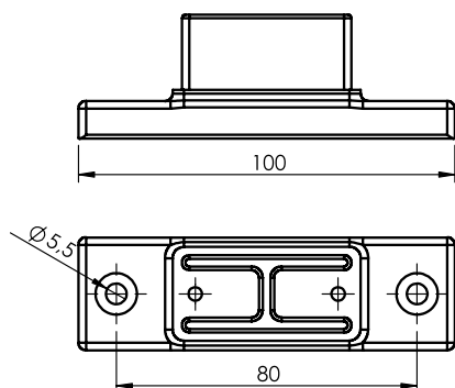
Patte de l'équerre élevée Av – Alu
