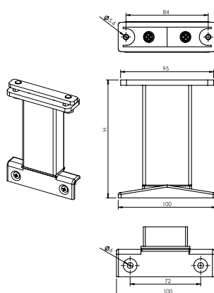
Équerre de coulisse VL Bv (2-01411-PU11X)
