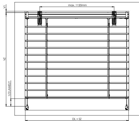
Guidage par cable - verticale
