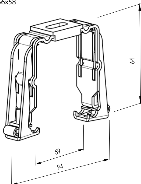
Etrier du boîtier - Fe Click P 002/32 (7-201862-0000) 56x58
