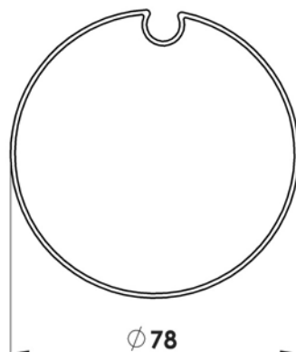
Tube d'enroulement (6-011084)
