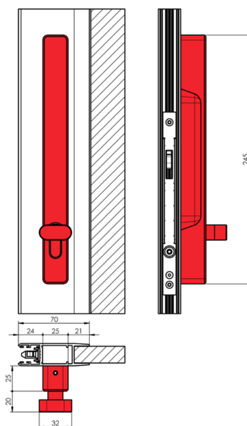
Poignée avec serrure, actionnée par un bouton
