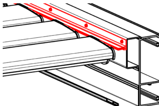
Petite brosse d'étanchéité côté non moteur
