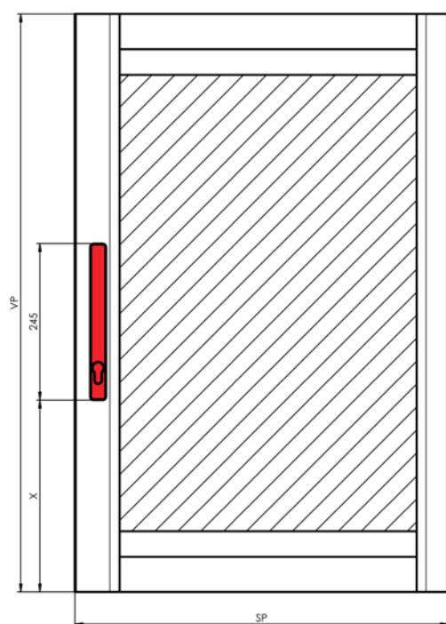
Poignée avec serrure, actionnée par une clé
